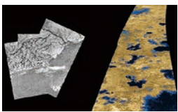
タイタンの地表にある川や湖 ©NASA
