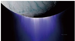
氷の割れ目から水蒸気を吹き出すエンケラドス ©NASA
