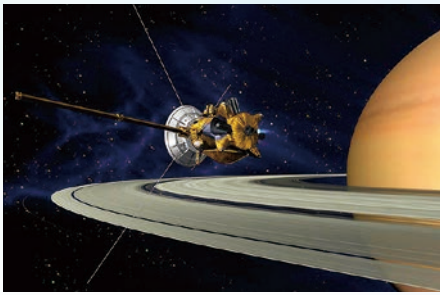
土星に到着したカッシーニ・ホイヘンス(想像図) ©NASA
