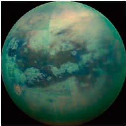
近赤外線撮影したタイタンの分厚い雲の下の様子 ©NASA
